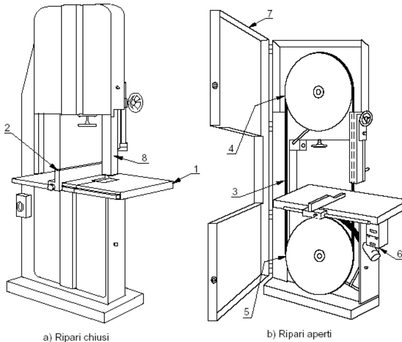
Terminologia per le seghe a nastro da falegnameria
